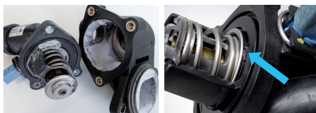
Figura 2: Los sellantes, los cuerpos extraños y los residuos provocan averías y bloqueos en el termostato
