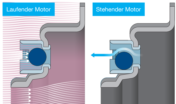
Abbildung 3: Bei laufendem Motor wird das Kugelventil durch das fließende Kühlmittel geschlossen
