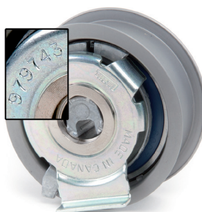
Figura 1: 531 0777 10 – versione precedente del rullo tenditore (979743)
