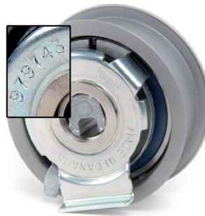
Photo 1: 531 0777 10 – Ancien galet tendeur (979743)
