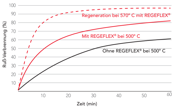
Filterregeneration mit und ohne REGEFLEX® (2L Euro 5 Motor/ 500° C)
