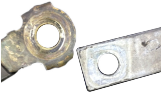
图示 1: 清洁前接地: 接触不良
